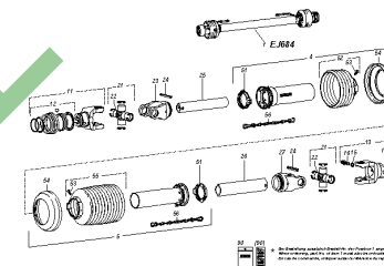
ETB-0000005673, Wałek przegubowo-teleskopowy EJ684 -W 100 E 710 mm, 1 3/8 cala, 6 sztuk
