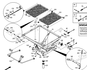
ETB-0000004621, Rama / zbiornik ZA-X 603
