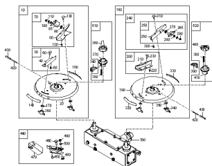
ETB-0000004638, Tarcza rozszewiająca
