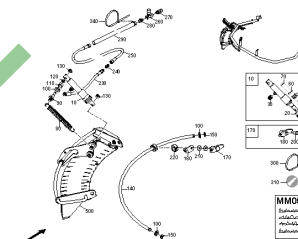
ETB-0000004723, Ekran rozsiewu granicznego - limiter, dołączony pakiet
