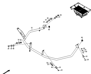
ETB-0000004624, Rurowy pałak ochronny ZA-X 903/1403
