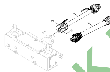
ETB-0000004710, Wałek przekąźnikowy
