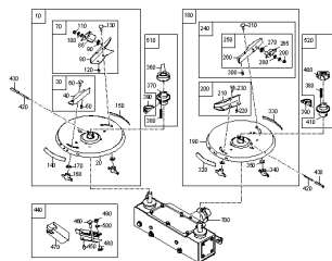
ETB-0000004638, Tarcza rozsiewająca
