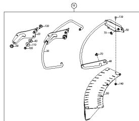
ETB-0000004719, Ekran rozsiewu granicznego - blacha prowadząca
