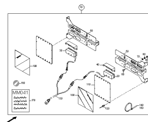
ETB-0000004747, Tylne oświetlenie ZA-X 603 / 1403
