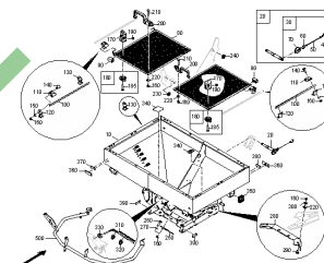
ETB-0000004632, Rama / zbiornik ZA-X 1403
