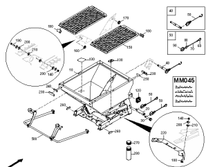
ETB-0000004614, Rama / zbiornik ZA-XW 503
