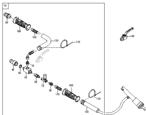
ETB-0000004661, Blok odcinający limitera
