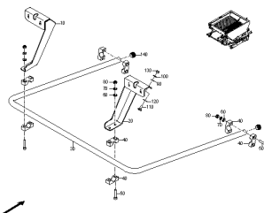
ETB-0000004620, Rurowy pałąk ochronny ZA-XW 503 / ZA-X 603
