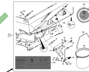
ETB-0000004734, Urządzenie do ustawiania odpowiedniej dawki rozsewu
