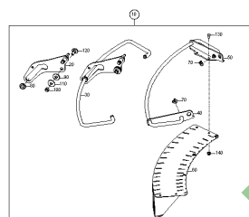
ETB-0000004719, Ekran rozsiewu granicznego - blacha prowadząca
