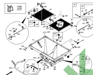
ETB-0000004623, Rama / zbiornik ZA-X 903
