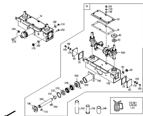
ETB-0000004702, Napęd mechaniczny / tarcze rozsiewające (1)
