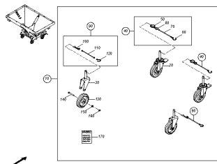
ETB-0000004708, Kółka transportowe hamowane
