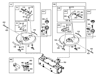
ETB-0000004638, Tarcza rozświetlająca
