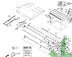
ETB-0000004743, Składana plandeka ZA-X 903 / 1403
