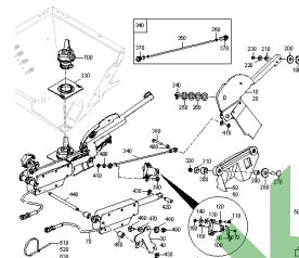
ETB-0000004687, Dno z otworami ZA-X Easy
