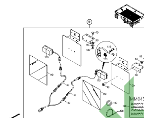
ETB-0000004774, Oświetlenie obrysowe przednie
