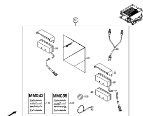
ETB-0000004746, Tylne oświetlenie ZA-XW 503
