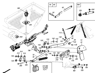
ETB-0000004666, Dno z otworami ZA-XW 503 / ZA-X 603
