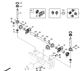
ETB-0000004705, Napęd mechaniczny / tarcze rozsiewające (2)
