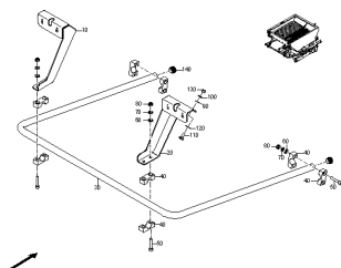
ETB-0000004620, Rurowy pałąk ochronny ZA-XW 503 / ZA-X 603
