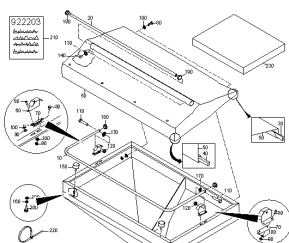
ETB-0000004766, Składana plandeka ZA-XW503 / ZA-X 603
