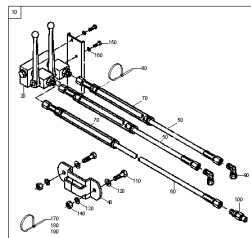
ETB-0000004671, Zespół dwudrogowy
