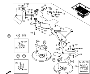
ETB-0000004731, Urządzenie do rozsiewu rzędowego do upraw owoców
