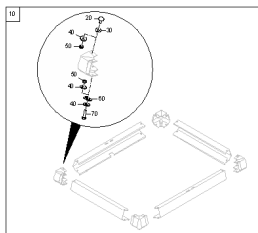
ETB-0000012432, Mocowanie elementów montażowych S203/S253
