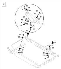
ETB-0000012430, Mocowanie elementów montażowych L1002/L803
