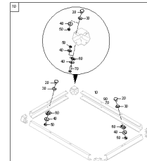
ETB-0000012428, Przystawka do elementów montażowych S353/S502
