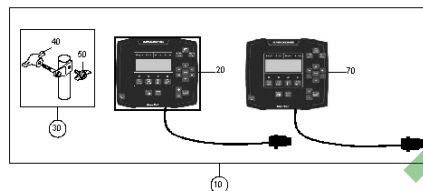
ETB-0000004745, Pakiet terminala Easy 2
