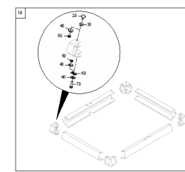
ETB-0000012432, Mocowanie elementów montażowych S203/S253
