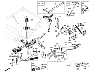
ETB-0000004681, Dno z otworami ZA-X 903/1403
