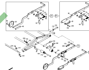
ETB-0000004744, Składana plandeka, dźwignia ręczna ZA-X 903 / 1403
