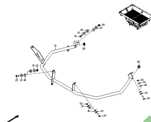
ETB-0000004624, Rurowy pałąk ochronny ZA-X 903/1403
