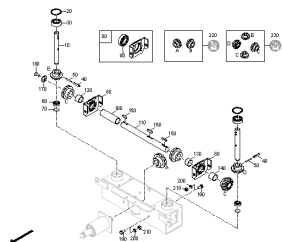
ETB-0000004705, Napęd mechaniczny / tarcze rozsiewające (2)
