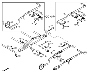
ETB-0000004744, Składana plandeka, dźwignia ręczna ZA-X 903 / 1403
